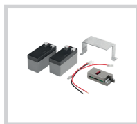
BRAINY24.CB Accesorio provisto de baterías CBY.24V, baterías 1,2 Ah y soporte.
